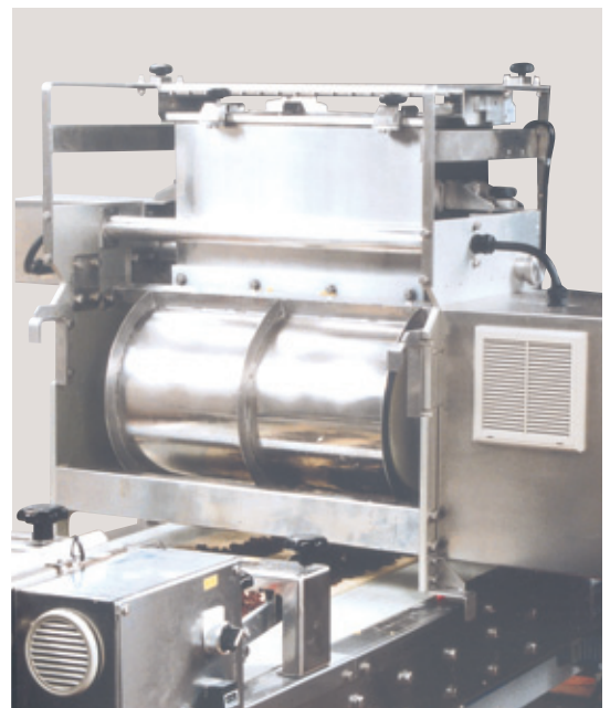
A：アジテータ（オプション）を付けることによって、粘着しやすい素材でも均一に吐出できます。
