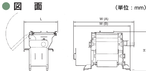
A：アジテータ（オプション）を付けることによって、粘着しやすい素材でも均一に吐出できます。
